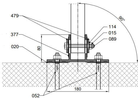
Snitt: Detalj a
