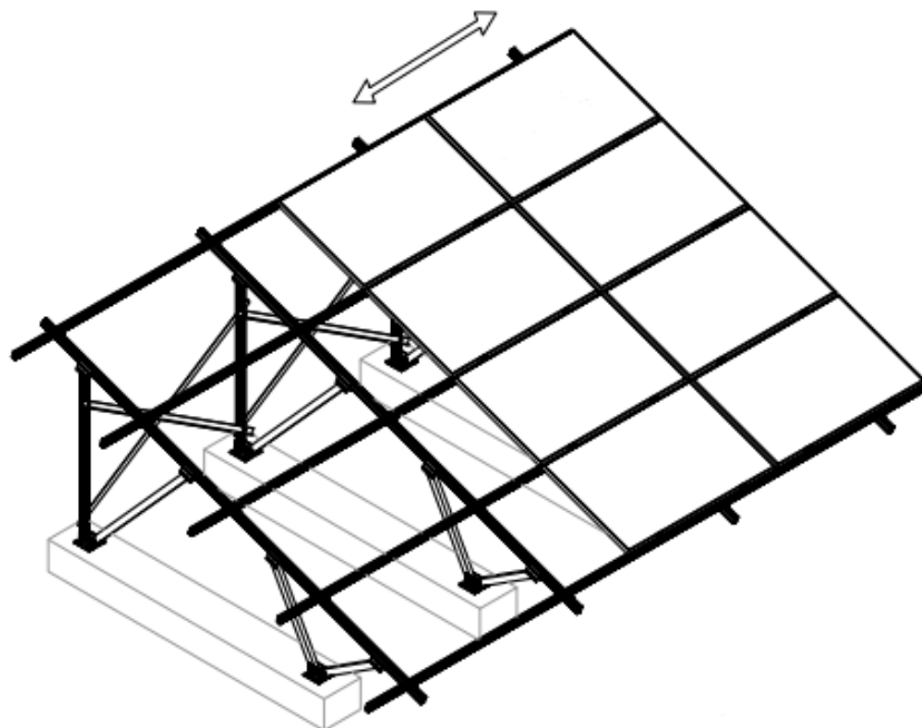
Horisontell montering av solpaneler
