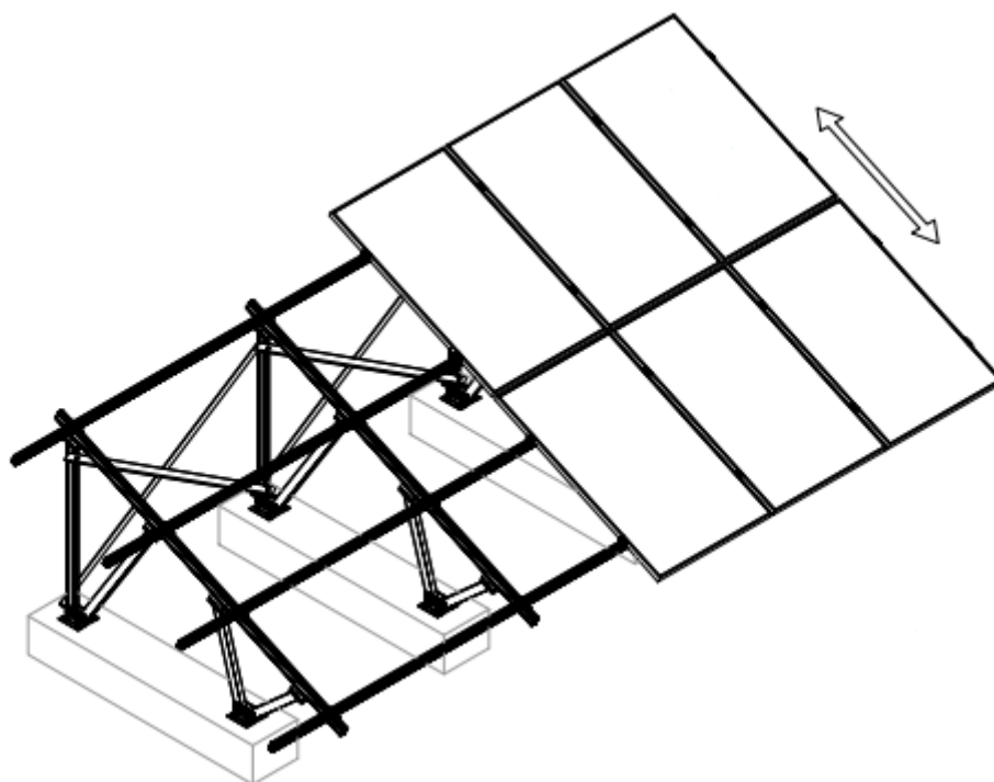
Vertikal montering av solpaneler
